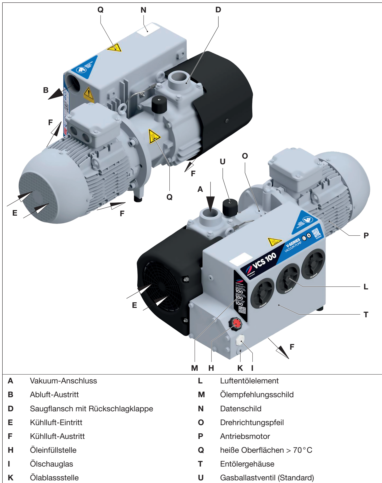
Abb. 2 Vakuumpumpe V-VCS 100 / 150
