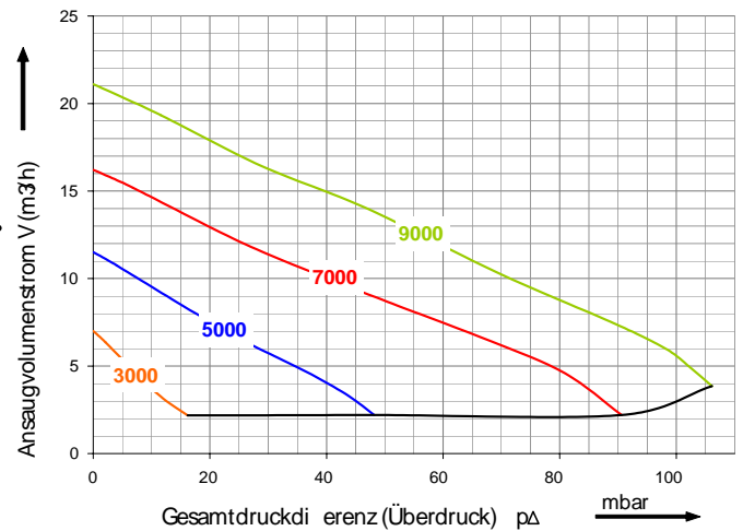
Kennlinie bei Betrieb als Kompressor, Überdruck
