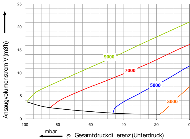
Kennlinie bei Betrieb als Vakuumpumpe, Unterdruck
